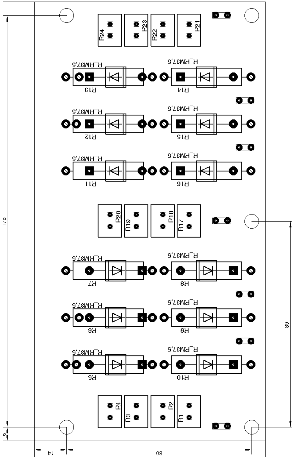
Bild 1: Anordnung/Mechanische Abmessungen
