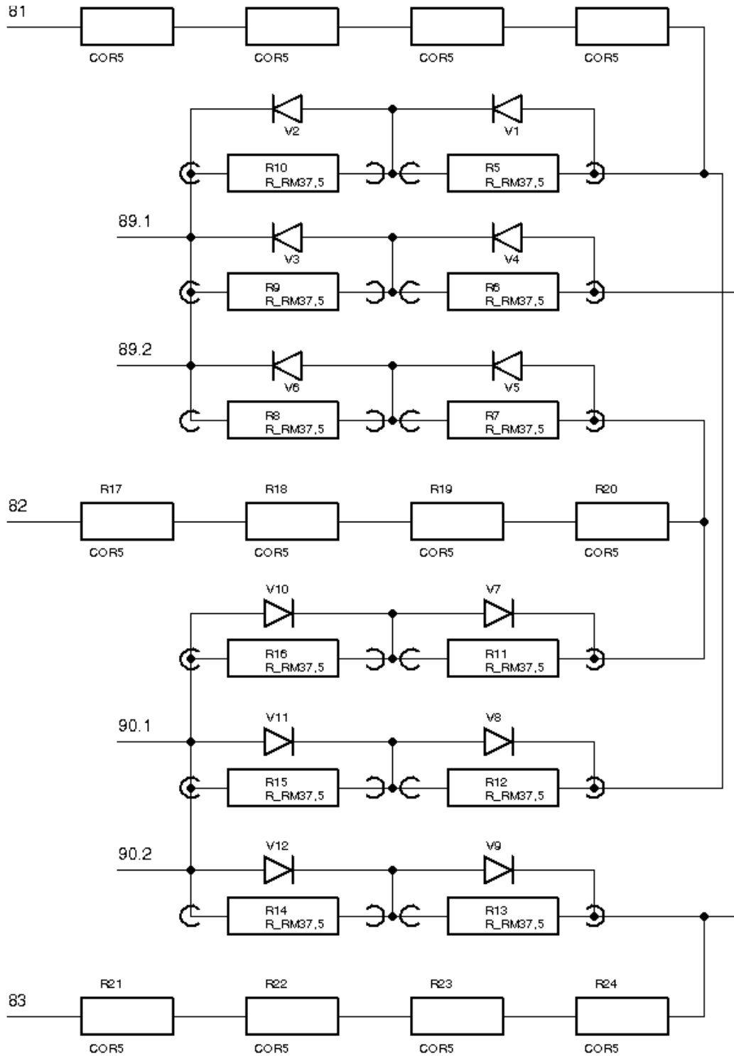
Bild 2: Schematik
